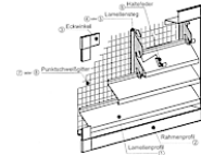
2. Lamellenbefestigung mittels Lamellenaufnahme
