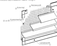
3. Lamellenbefestigung mittels Schrauben bzw. Nägel
