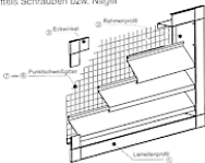
3. Lamellenbefestigung mittels Schrauben bzw. Nägel
